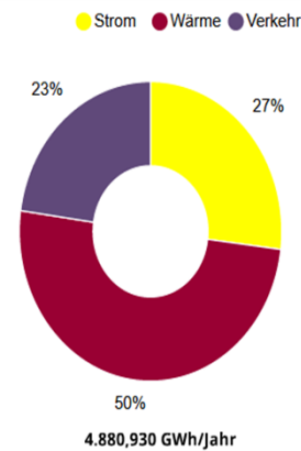
Endenergieverbrauch gesamt 2019
