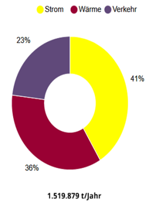
Treibhausgasemissionen (CO 2 -Äquivalente) gesamt 2019
