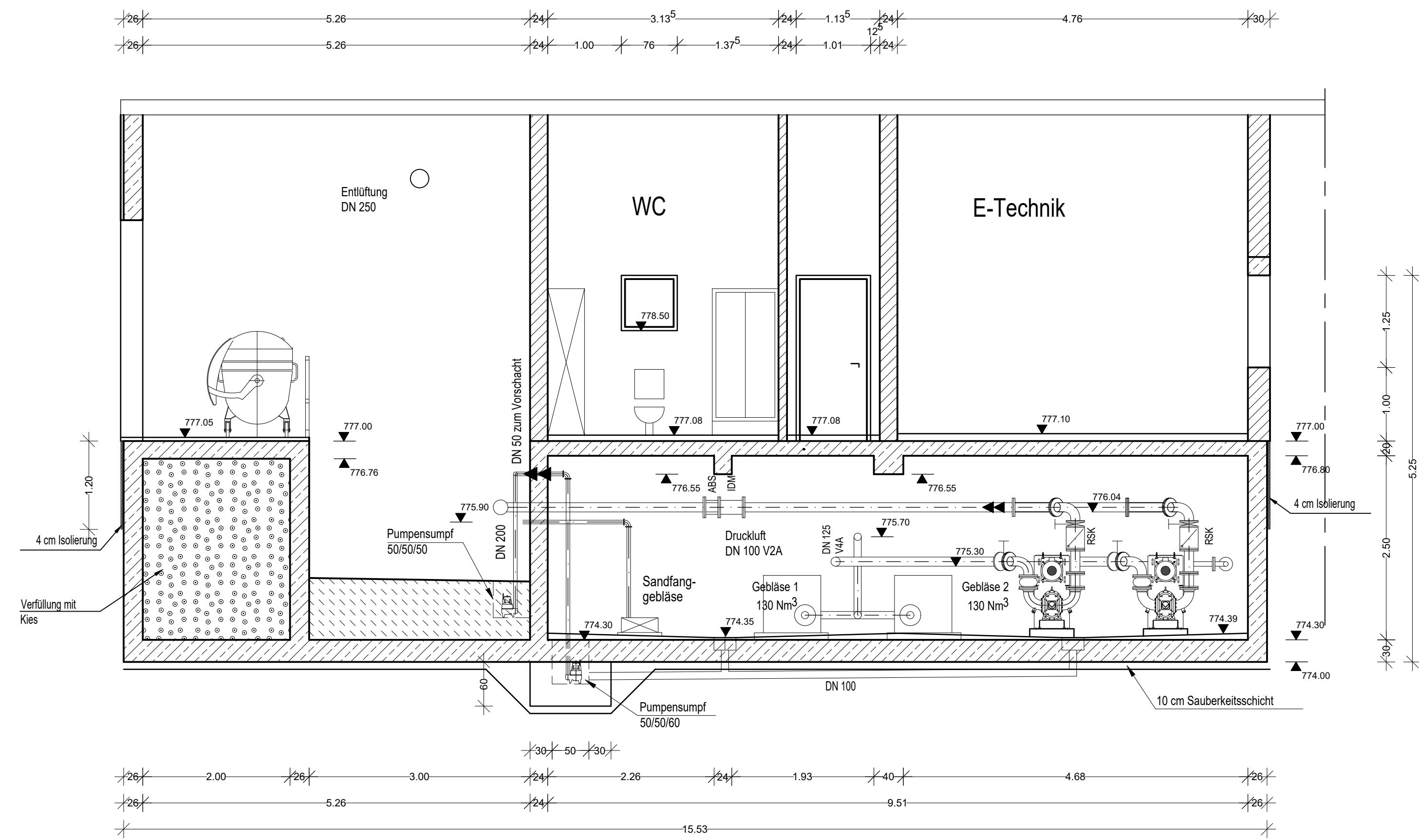
Schnitt P - P
