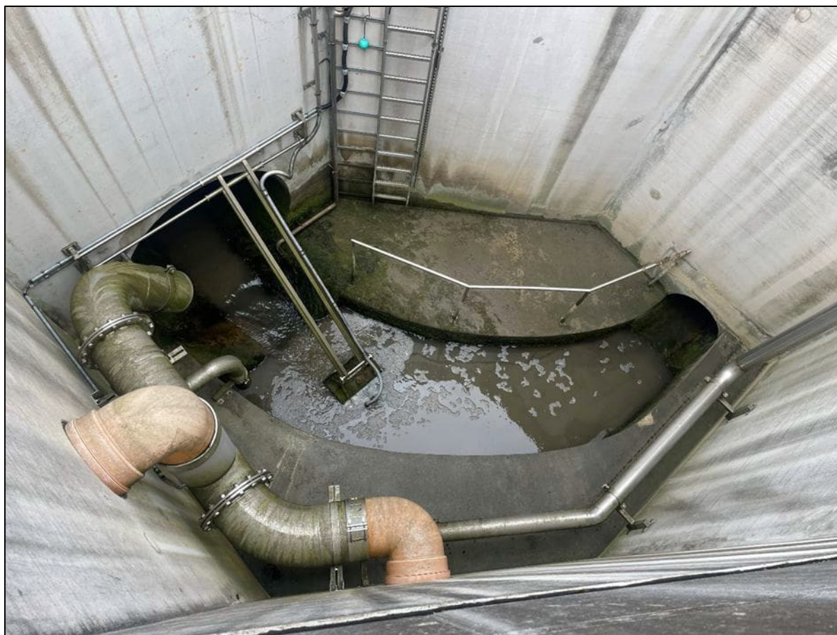
Abbildung 2: Analyseschacht (Schacht R41/11)
